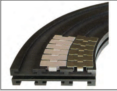
Profil Bölümü/Profiles: "C" L= 82,6 P= 84 mm
