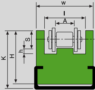
Profil Bölümü/Profiles: "UCC"
