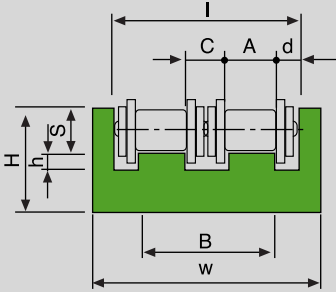
Profil Bölümü/Profiles: "UCD"
