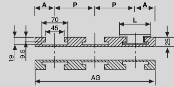
Profil Bölümü/Profiles: "C" L= 82,6 P= 85 mm
